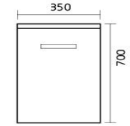
▲ TB - 09D 1 Door Cabinet
