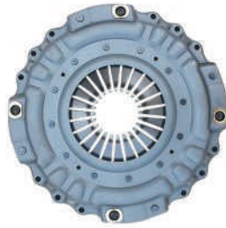
品名: EQ430膜片式盖总成 规格: 430*228*450 适配车型: 东风康明斯6CT 奔驰 大金龙 宇通 Product Name:EQ430 diaphragm type cover assembly Specification:430*228*450 Fit models:Dongfeng Cummins 6CT Yutong Benz Jinlong
