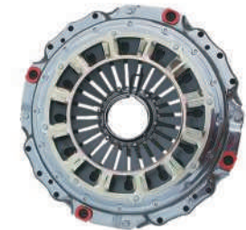
品名: 拉式430大孔盖总成 规格: 430*235*450 适配车型: 斯太尔王 豪沃 奥龙 Product Name: Pull type 430 big cover assembly Specification:430*235*450 Fit models:Steyr HOWO oron
