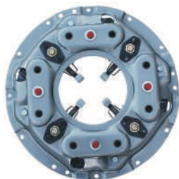
品名: 430周置式盖总成 规格: 430*250*456 适配车型: 五十铃 三菱 Product Name: 430 weeks of floating cover assembly Specification:430*250*456 Fit models:Isuzu Mitsubishi
