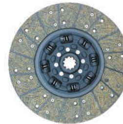
品名: EQ145从动盘总成 规格: 350*216*10*38.4 适配车型: 玉柴6112 ELQ机 YC6108 Product Name:EQ145 driven disc assembly Specification:350*216*10*38.4 Fit models:Yuchai 6112 ELQ Yc6108
