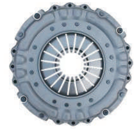
品名: 膜片式395盖总成 规格: 395*215*410 适配车型: 东风康明斯 Eq395 Product Name:Explosion proof type 395 cover assembly Specification:395*215*410 Fit models:Dongfeng Cummins EQ395
