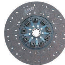
品名: 拉式430从动盘总成 规格: 430*240*10*50.8 适配车型: 新大威 斯太尔王 豪沃 奥龙 Product Name: Pull the 430 driven disc assembly Specification: 430*240*10*50.8 Fit models: New Venus Steyr HOWO oron
