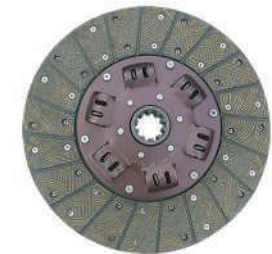
品名: EQ140从动盘总成 规格: 325*190*10*38.4 适配车型: EQ140D2 EQ1090YC6105 CY6102 Product Name:Pull the 430 driven disc assembly Specification:325*190*10*38.4 Fit models:EQ140D2 EQ1090 YC6105 CY6102
