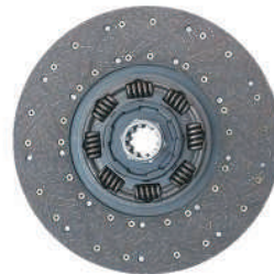
品名: 拉式430从动盘总成 规格: 430*230*10*44.55 适配车型: 金龙大客 斯塔尼亚 Product Name: Pull the 430 driven disc assembly Specification: 430*230*10*44.55 Fit models: Jinlong Passenger staneyr
