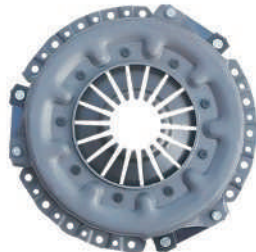
品名: 255高齿膜片式盖总成 规格: 255*160*290 适配车型: 北京BJ1041 4102Q 492Q YN4100Q Product Name: Φ255 diaphragm type cover assembly Specification:255*160*290 Fit models:BJ1041 4102Q 492Q YN4100Q
