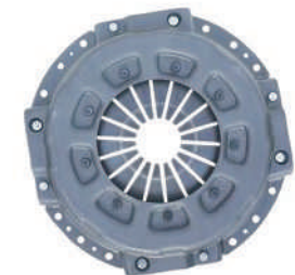
品名: Φ275膜片式盖总成 规格: 275*178*320 适配车型: EQ1060/1061 江淮 郑州东风 Product Name:Φ275 diaphragm type cover assembly Specification:275*178*320 Fit models:EQ1060/1061 JAC zhengzhou DFM
