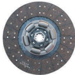
品名: EQ395从动盘总成 规格: 395*230*10*44.55 适配车型: 东风康明斯 EQ395 Product Name:EQ395 driven disc assembly Specification:395*230*10*44.55 Fit models:Dongfeng Cummins Eq395
