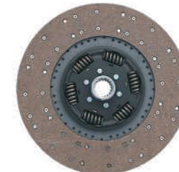
PartNo:3482 000 634 Type No:MF395 Size:395*235*410
