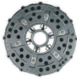
品名: 420螺旋式铸铁盖总成 规格: 420*215*450 适配车型: 道依茨 Product Name:420 spiral iron cover assembly Specification:420*215*450 Fit models:Deutz
