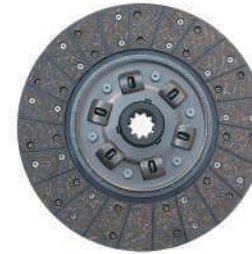
品名: CA151从动盘总成 规格: 350*216*10*38.4 适配车型: 玉柴6112 ELQ机 YC6108 Product Name:CA151 driven disc assembly Specification:350*216*10*38.4 Fit models:FAW Jie Fang Ca151
