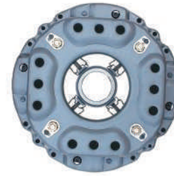
品名: 防爆式395盖总成 规格: 395*215*410 适配车型: 东风康明斯 EQ395 Product Name:Explosion proof type 395 cover assembly Specification:395*215*410 Fit models:Dongfeng Cummins EQ395
