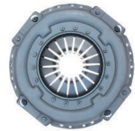
品名: EQ153膜片式盖总成 规格: 380*200*410 适配车型: 东风康明斯 Product Name:EQ153 diaphragm type cover assembly Specification:380*200*410 Fit models:Dongfeng Cummins
