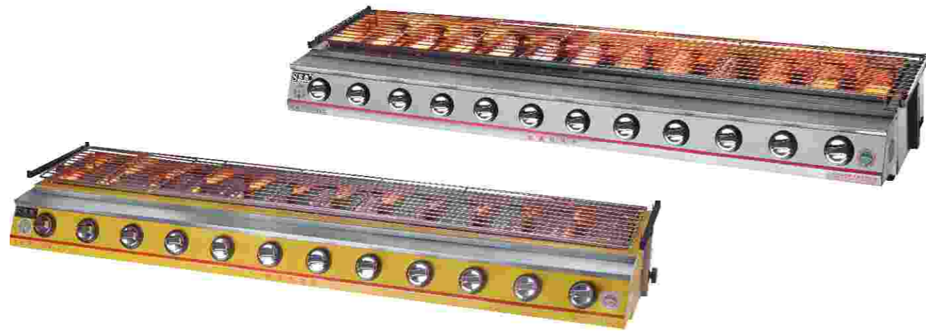
名称Name: 十二头环保烧烤炉Gas BBQ Grill 型号Model: SC-SR12G SC-SR12 SC-SR122 SC-SR122B 颜色Color: 不锈钢 不锈钢 黄色 黄色 配置Configuration: 不锈钢罩 耐高温玻璃罩 不锈钢罩 耐高温玻璃罩 规格Dimension: 1500x425x200mm 净重N/W: 25kg 气压Pressure: 2800pa (液化石油气, 可定做天然气) 烧烤面积Grill size: 1480x250mm
