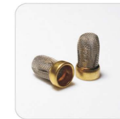
BC5509B ASNU03W VW Nippondenso, Multec, GM \phi 6.08 \times 3 \times 10.3\text{mm}
