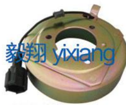
YX17187 名称 /Car Make: 尺寸 /Size: 104.8x66.5x28x40mm
