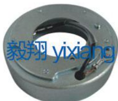
YX17145 名称 /Car Make: 96 尺寸 /Size: 85x55x23.5x40mm
