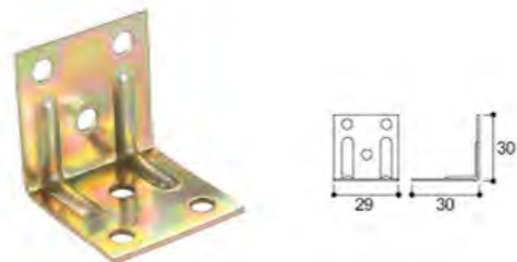
品名：角码 Name：Angle piece
