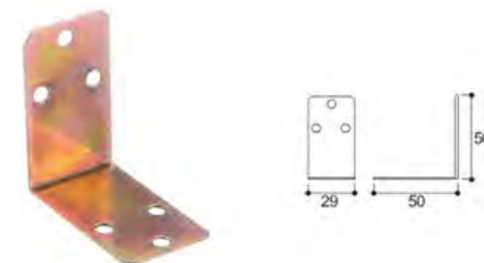
品名：连接角码 Name：Connecting bracket
