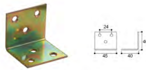
品名：角码 Name：Angle piece
