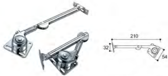
品名：液压支撑器 Name: Hydraulic stay
