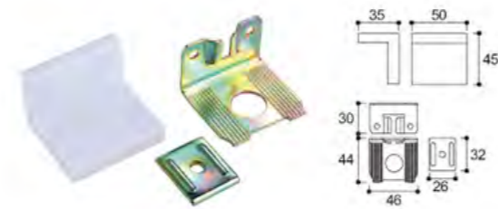
品名：角码 Name：Angle piece
