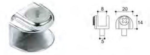
品名：玻璃夹 Name: Glass clip TG074
