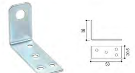
品名：角码 Name：Angle piece
